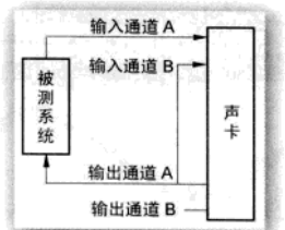
图8 频率响应测试连线图
