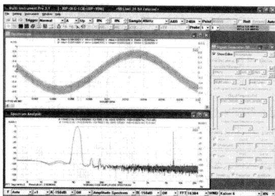
图5 声卡自身的IMD测量
