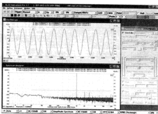
图4 声卡自身的THD、THD+N、SINAD、SNR、NL测量
