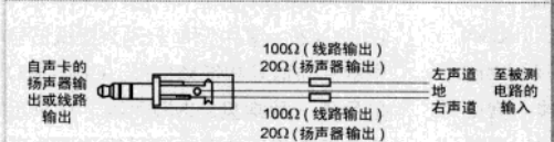
图3 具有简单短路保护的输出连接方式
