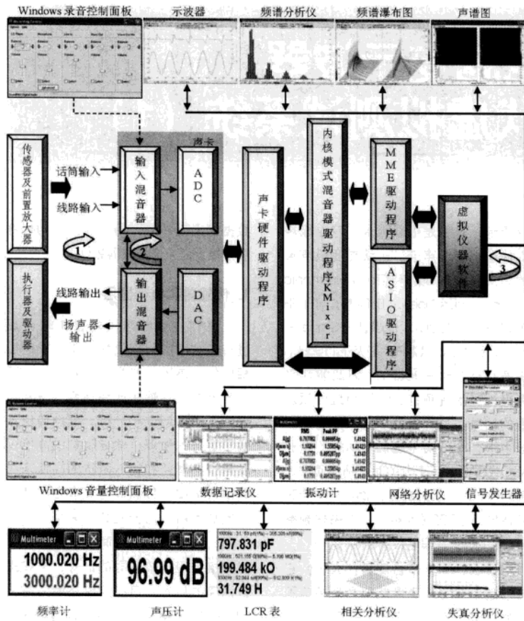
基于声卡的测试系统的基本架构
