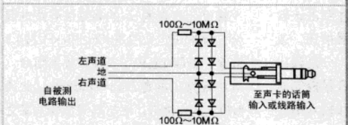
图2 具有简单过压保护的输入连接方式
